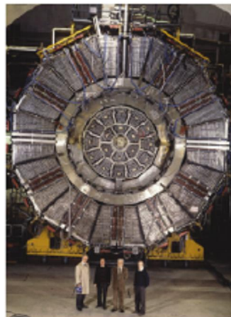
EL DETECTOR ALPHA JUNTO A SUS CREADORES. EN EL CILINDRO CENTRAL TIENEN LUGAR LAS COLISIONES QUE SE REGISTRAN A TRAVÉS DE SENSORES EN SUS PAREDES.
